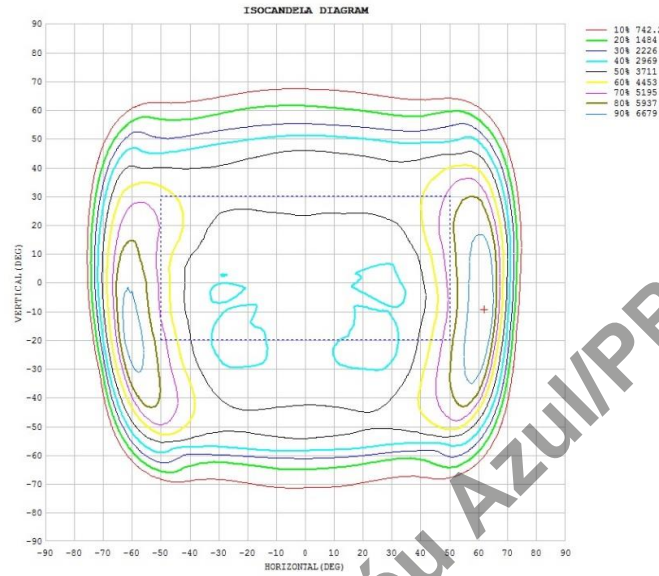
Figura 3 - Curva de distribuição de intensidade (isocandela) (51241-1).
