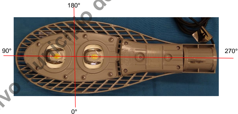
Foto 4 - Eixos Fotométricos
